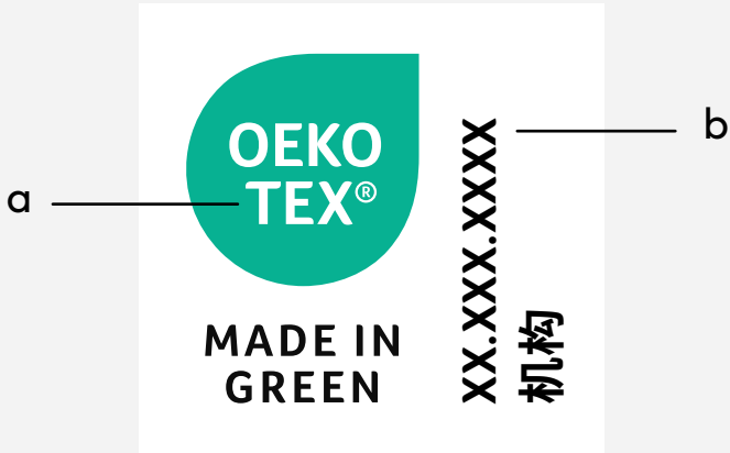
强制元素：
